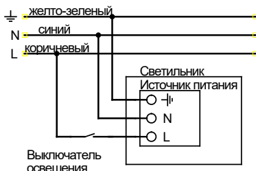
Рис.1. Схема подключения
