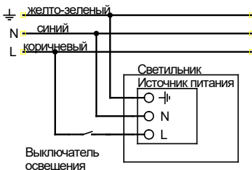
Рис.1. Схема подключения
